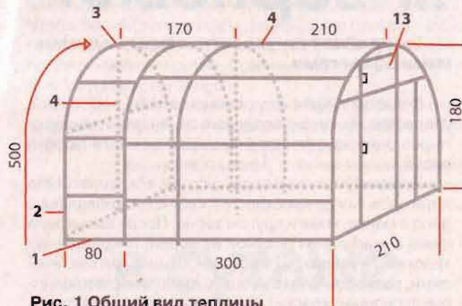
Рис. 1 Общий вид теплицы
