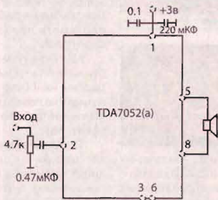
Принципиальная схема
